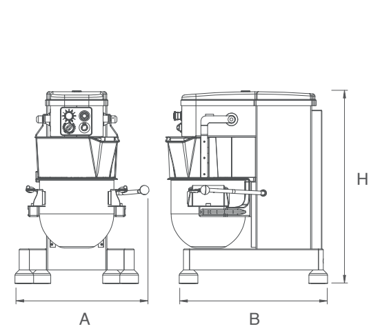
Dessins techniques C-Line 2 10/20 – sur table
